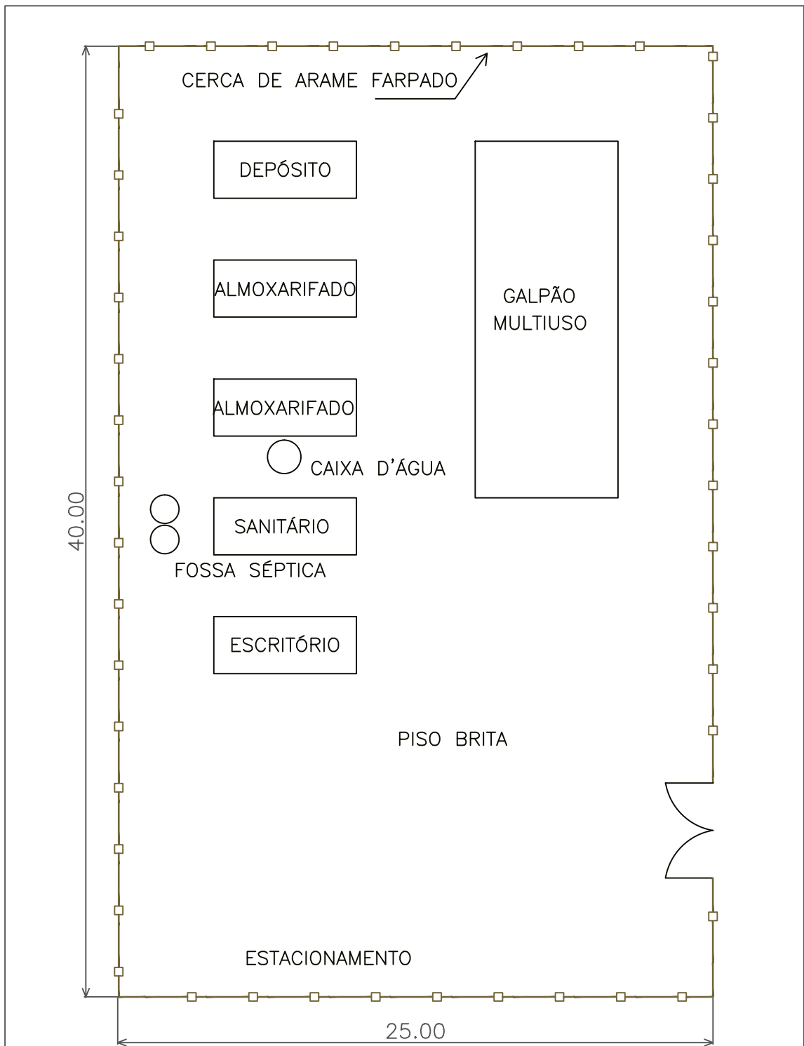
PLANTA ESCALA 1:200
